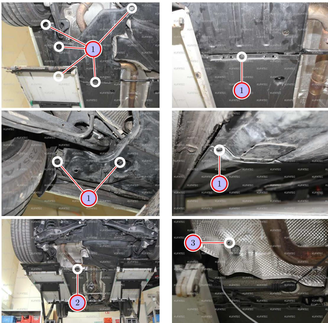
Abbildung 9: Verlegung Anschlusskabel Geräuscherzeuger Unterboden
