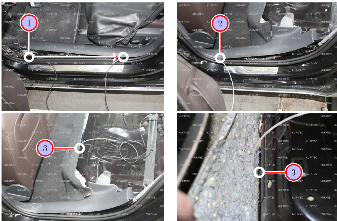
Abbildung 8: Verlegung Anschlusskabel Geräuscherzeuger
