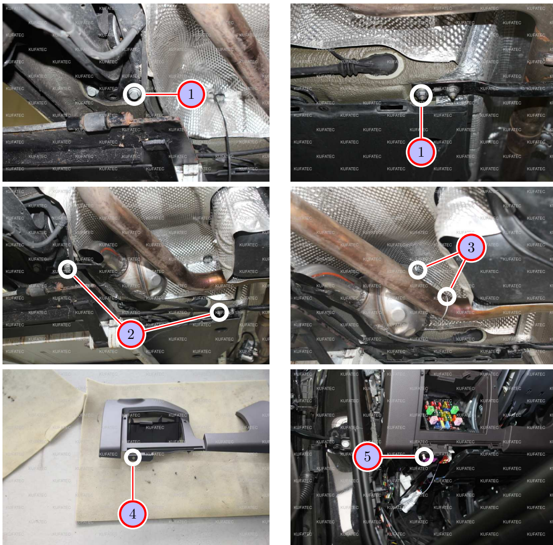
Abbildung 10: Montage Geräuscherzeuger / Taster
